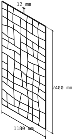
Isométrico · 12 mm
