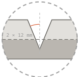
24 mm V 22.5° · baja 18 mm boca 14.91 mm
