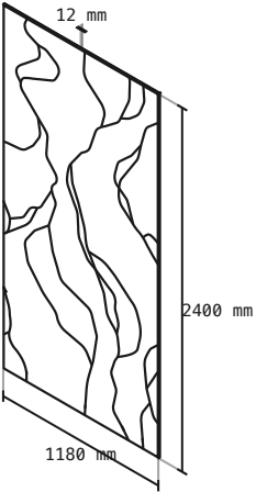
Isométrico · 12 mm
