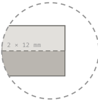
24 mm canto recto · sin bisel 2 láminas · 1.28 kg/m
