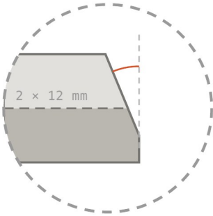
24 mm V 22.5° · baja 18 mm junta: boca 14.91 mm
