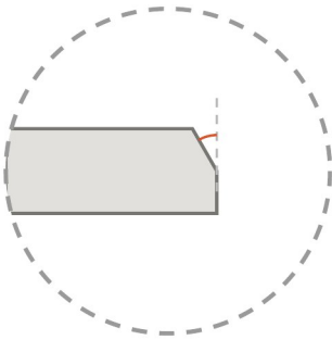
12 mm V 30° · baja 6 mm junta: boca 6.93 mm
