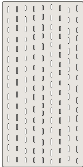
PAREJO 146 calados · 6.9 % abierto
