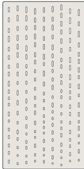
ARRIBA 173 calados · 5.5 % abierto
