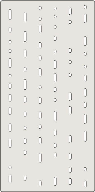
BAMBÚ Parejo · paso 180 — 74 calados · 5.4 % abierto
