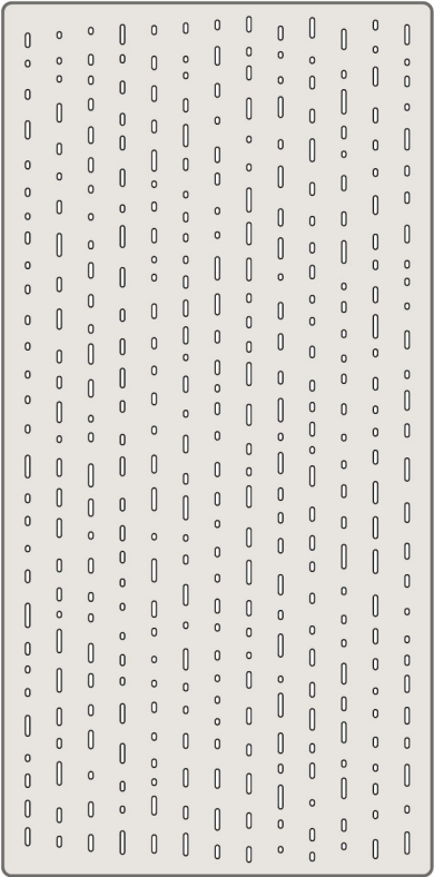
LLUVIA Arriba · paso 90 — 374 calados · 5.2 % abierto
