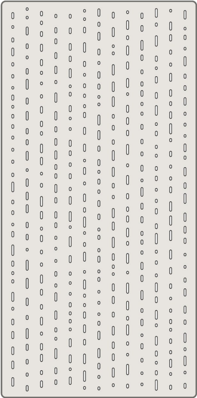
ALTA paso 86 mm — 390 calados · 5.1 % abierto
