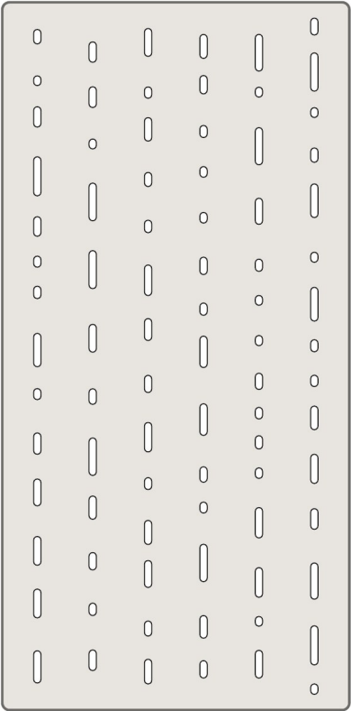
BAJA paso 180 mm — 84 calados · 4.9 % abierto
