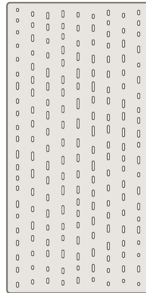
CENTRO 179 calados · 5.4 % abierto
