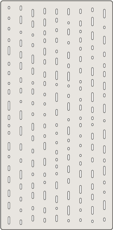
MEDIA paso 130 mm — 177 calados · 5.4 % abierto
