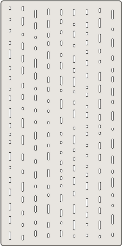
JUNCOS Abajo · paso 130 — 177 calados · 5.4 % abierto
