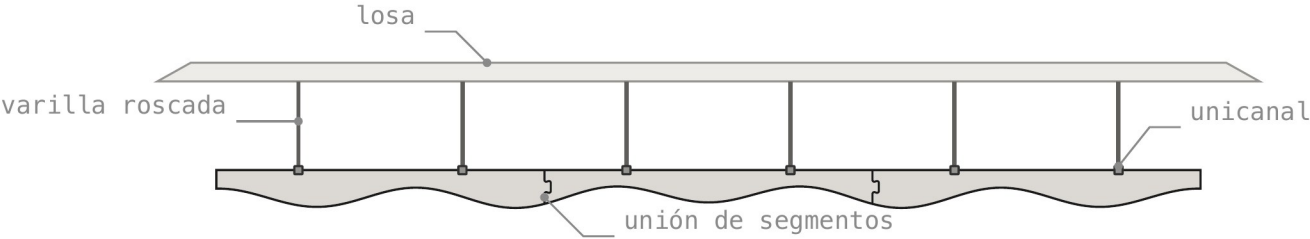
DETALLE DEL HERRAJE
