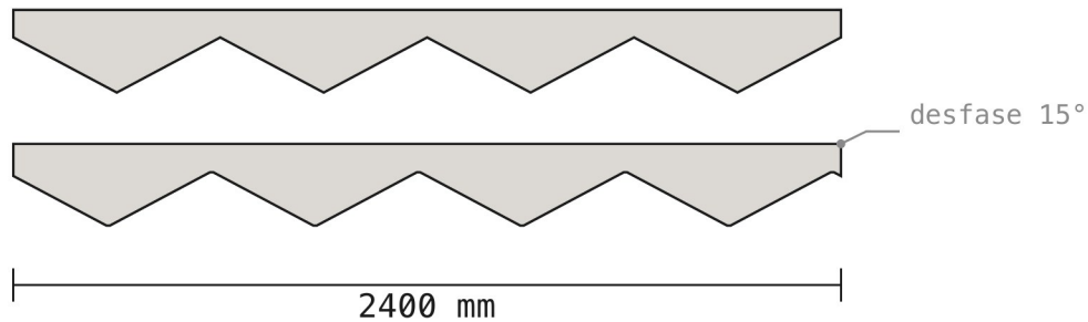
DOS BAFLES CONSECUTIVOS • A ESCALA
